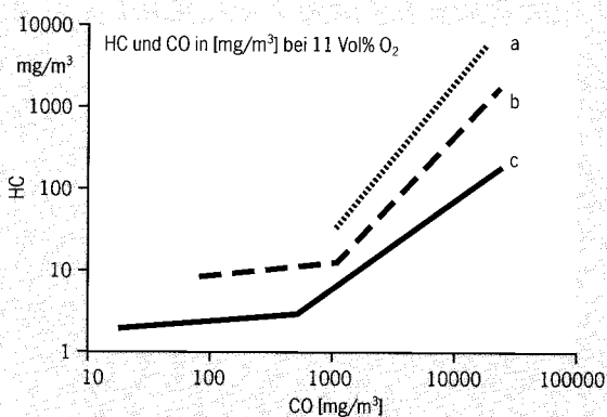
Abbildung 5: Korrelation zwischen Kohlenwasserstoff-(HC) und Kohlenmonoxidemissionen (CO) bei Holzfeuerungen: a) Kamin mit Sichtfenster, b) Stückholzkessel mit unterem Abbrand, c) Untersubfeuerungen, [22].
