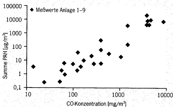
Abbildung 4: Korrelation zwischen PAK- und Kohlenmonoxidemissionen bei Verbrennung von Holz-schnitzeln, Rinde, Spänen und Spanplatten in Stückholz-, Untersub- und Rostfeuerungen [21]
