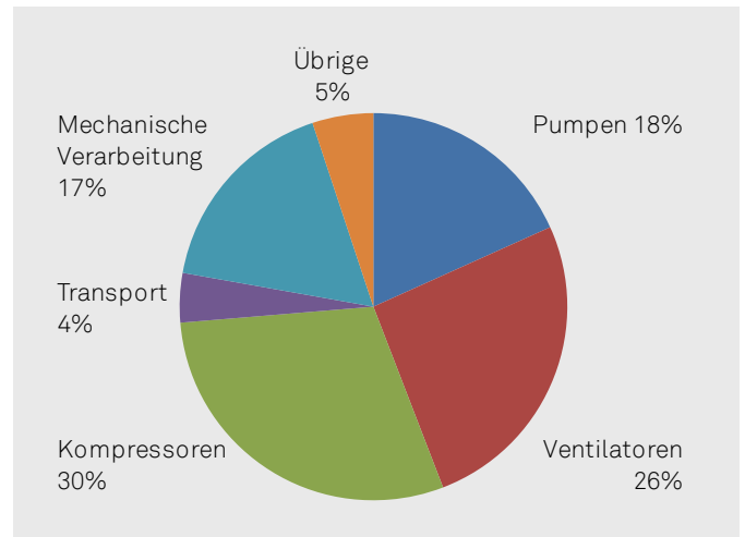
Abbildung 2: Anwendungen von elektrischen Motoren bei 5 grossen Industrieunternehmen (Quelle: Easy 2012)
